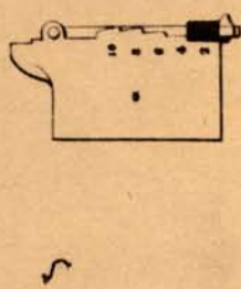
Fig 6. Hausse montée.
