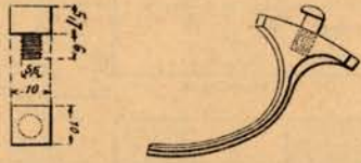
Fig. 3. Pontet du Revolver M le 1873 Remplacement du T. (1/2).
