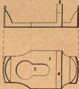
Fig 15 Verrou d'anneau de calotte
