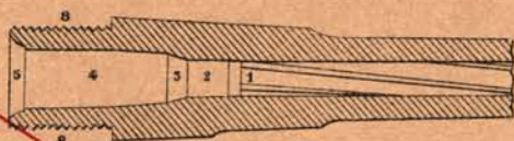
Fig.3. Coupe longitudinale.
