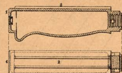
Fig. 8. Poignée.
