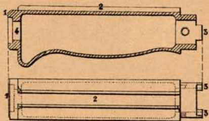
Fig. 6. Poignée.
