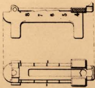
Fig 2 Hausse montée.
