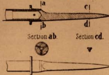
Fig 2 ter Monture de la partie antérieure de la lance ( \frac{1}{4} ).
