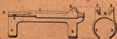
Fig 3 Pied de hausse à griffes.
