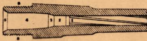
Fig 3. Coupe longitudinale
