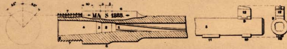
Fig 2 Vue du côté droit
