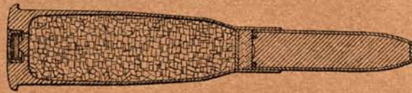
Fig.7. Coupe de la. Cartouche M le 1886M.
