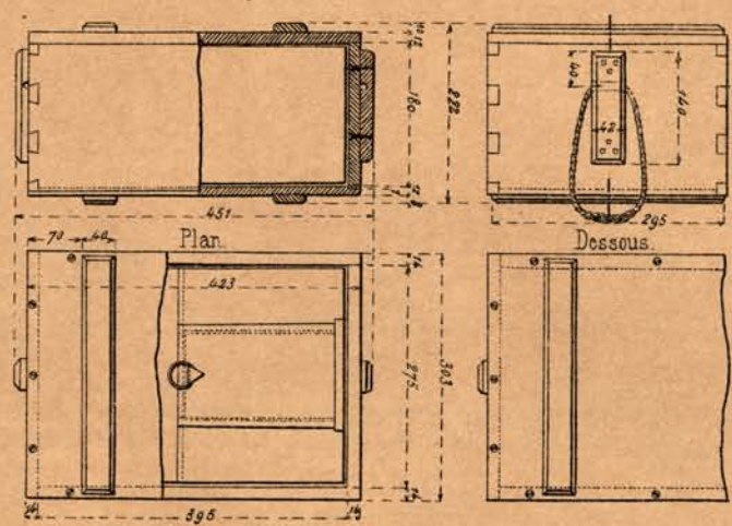
Fig. 9. Caisse C.2 bis avec caisse intérieure en zinc. Elevation et coupe longitudinale. Vue de bout.
