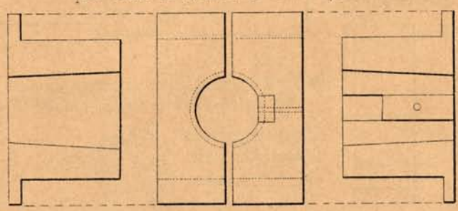
Fig. 3. Presse à semelle. ( \frac{1}{4} )
