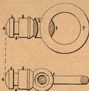
Fig 14 Anneau de calotte et son pivot
