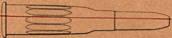
Fig.4 Fausse cartouche M le 1892.
