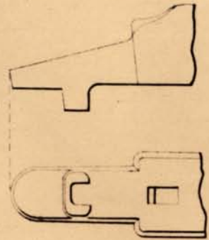
Fig 11 Tenon de recul de la boîte de culasse.
