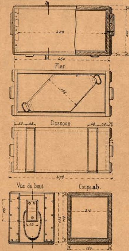
Planchette de la caisse M 1 e T.
