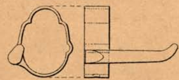
Fig 13 bis . Embouchoir à quillon pour mousqueton M le 1902.
