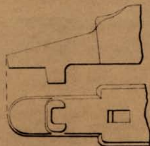
Fig. 11. Tenon de recul de la boîte de cuisse.
