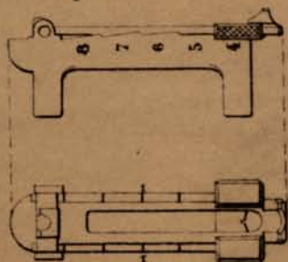
Fig. 2. Hausse montée.
