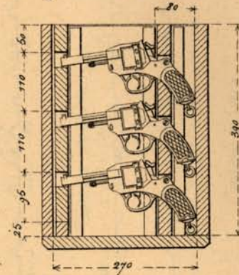
Fig. 3. Caisse disposée pour les M les 1892 et 1874. Coupes suivant ABC.
