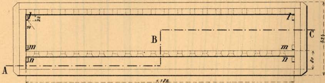
Tasseau intermédiaire de poignées. ( \frac{1}{5} ).
