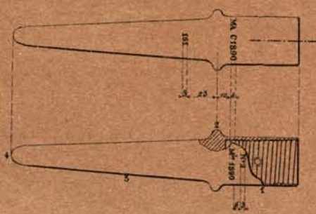
Fig 5 Sabot ( \frac{1}{4} ).
