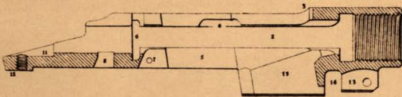
Fig 14. Coupe longitudinale.
