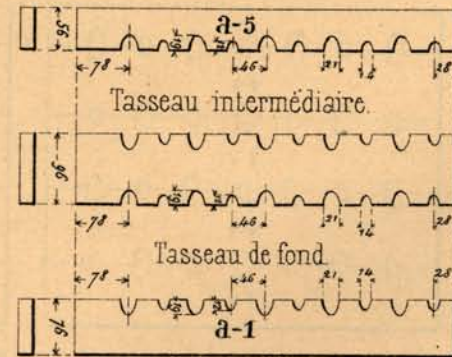
Tasseau de dessus.
