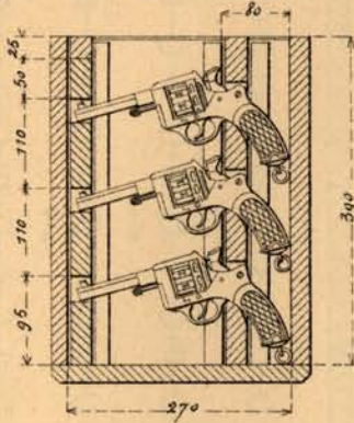
Fig. 3. Caisse disposée pour les M les 1892 et 1874. Coupes suivant ABC.
