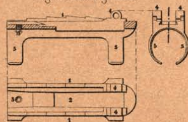
Fig. 7. Pied à griffes.
