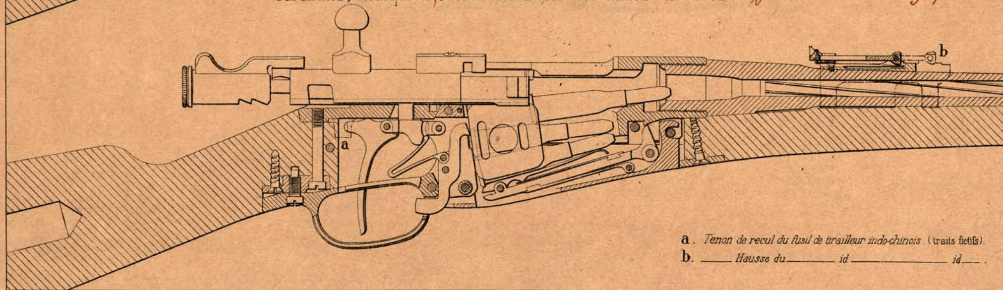
Carabines, Mousqueton, et fusil de traillleur indo-chinois. M le 1902 et fusil colonial M le 1907
