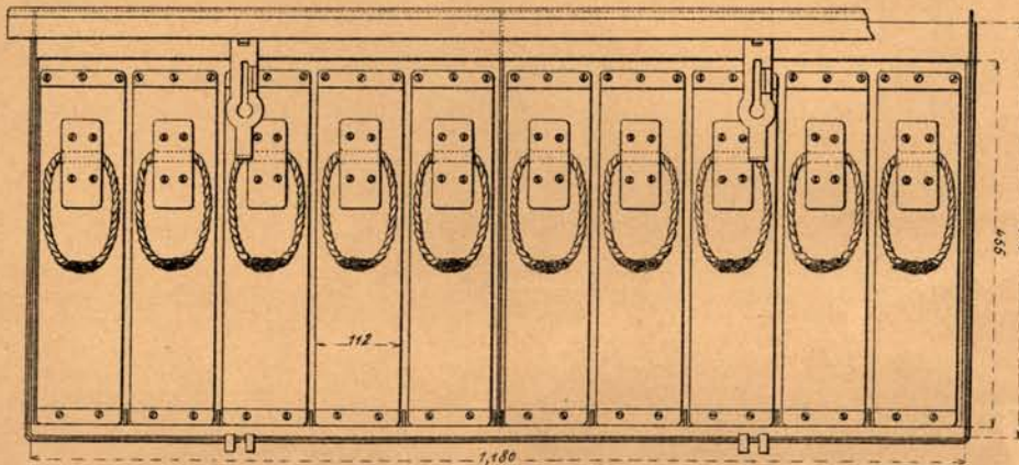
Caisse à munitions de montagne M le 1862.
