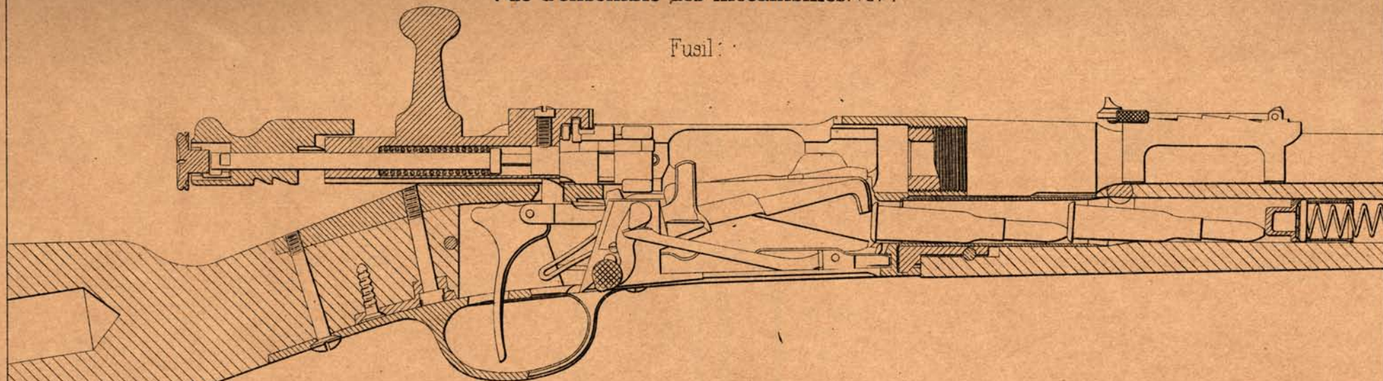
Carabines, Mousqueton, et fusil de traillleur indo-chinois. M le 1902 et fusil colonial M le 1907
