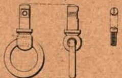
Fig 8. Anneau de calotte. Pivot d'anneau de calotte et sa vis.
