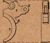
Fig 13. Détente.
