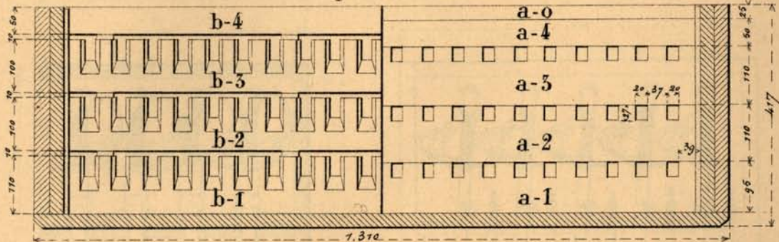
Fig. 3. Caisse disposée pour les M les 1892 et 1874. Coupes suivant ABC.
