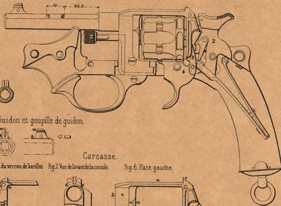
Fig.2 Vue du côté gauche, la platine à découvert.
