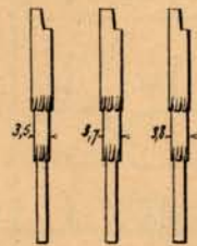
Fig. 5. Fraises à rectifier les trous de poignée. (1/2).
