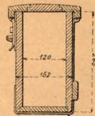
Fig. 8. Coupe gh.
