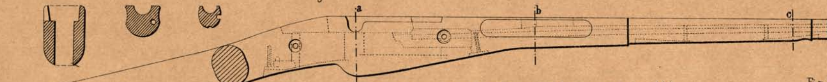
Monture de carabine de cavalerie. ( \frac{1}{4} ).
