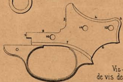
Fig.9. Vue extérieure.
