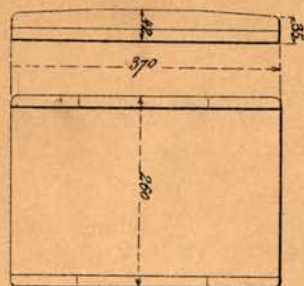
Fig. 3. Planche de pression.
