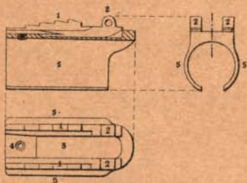
Fig.5. Pied de hausse.
