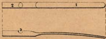
Fig.9 Ressort d'axe de barillet.
