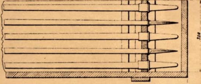
Chargement en lances M le 1913.
