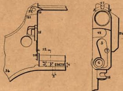
Fig.5. Logement du verrou de barillet Fig.7. Vue de l'avant de la console.
