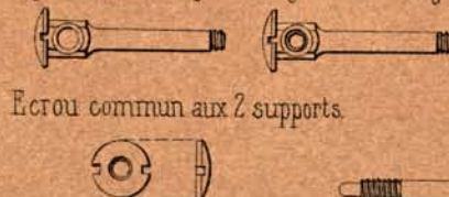
Fig 14. Guide de baguette. Fig 15. Ecrrou de baguette.
