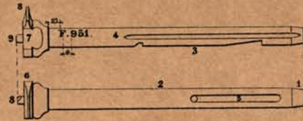
Fig 2. Axe du barillet.
