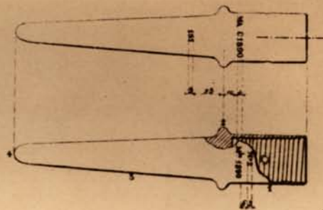
Fig 5 Sabot ( \frac{1}{4} ).
