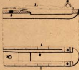
Fig 16 Coupe de la queue de culasse M le 1886.
