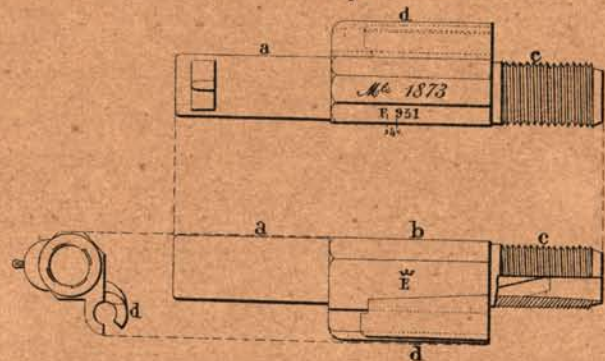
Fig 3. Canon.
