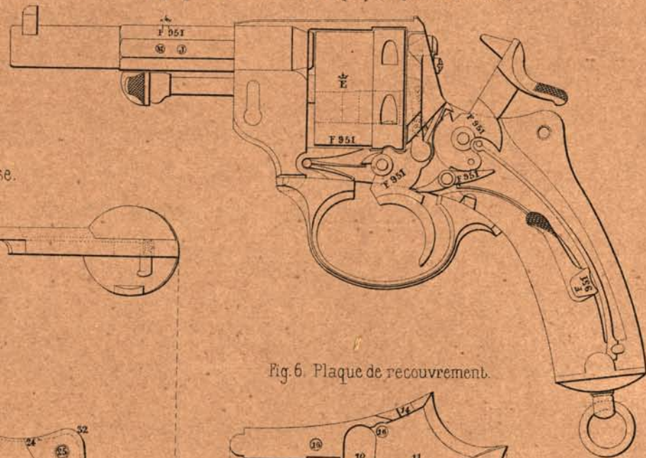
Fig 2 Vue d'ensemble du mécanisme. (la plaque de recouvrement et la plaquette gauche enlevées).
