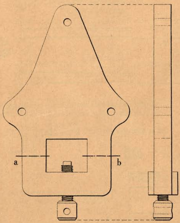
Fig. 6. Déculassage d'une carabine ou d'un mousqueton.
