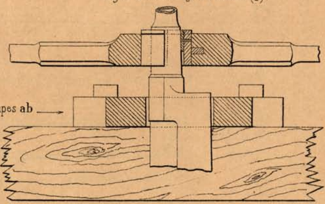
Fig. 7. Déculassage d'un fusil. ( \frac{1}{2} )
