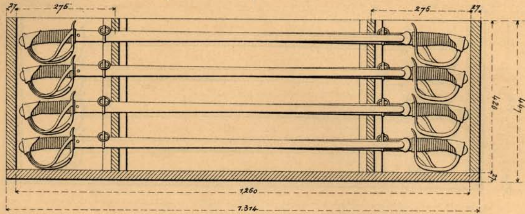
Coupe montrant la disposition des armes.
