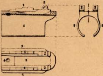
Fig 5. Pied de hausse.
