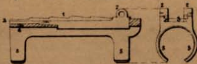
Fig. 4. Ressort de hausse.
