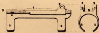
Fig 3 Pied de hausse à griffes.
