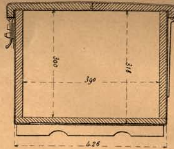
Coffre de caisson léger à munitions d'infanterie.
