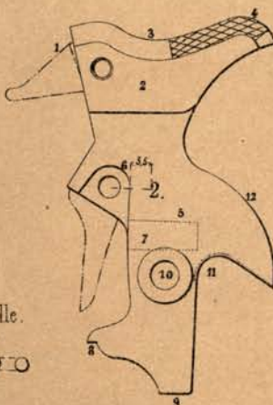
Fig 14 Anneau de calotte et son pivot
