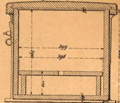
Fig. 5. Coupe ab
