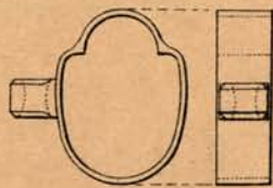
Fig 12. Grenadière.
