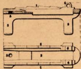
Fig 7 Pied à griffes
