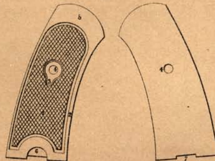
Fig 17 Plaquette gauche (1/2)
