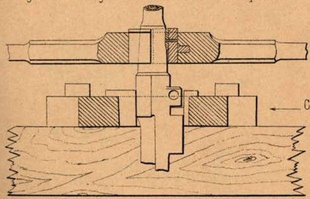
Fig. 6. Déculassage d'une carabine ou d'un mousqueton.
