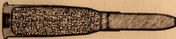
Fig. 7. Coupe de la Cartouche M le 1886 M.
