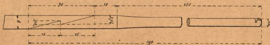
Fig.7. Baguette de nettoyage. (+).
