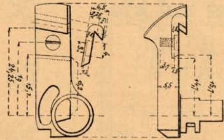
Fig. 9. Pièce rapportée à l'épaule- ment d'arrêt de la porte. (1/2).
