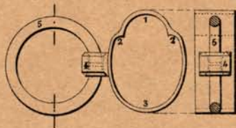
Fig. 14. Grenadière. (à anneau).
