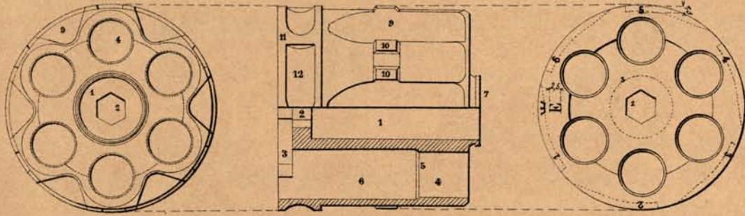
Fig.2. Extracteur.
