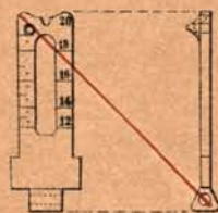
Fig.7. Plaque de hausse.
