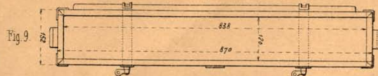
Plan de la caisse et de la planchette de remplissage.
