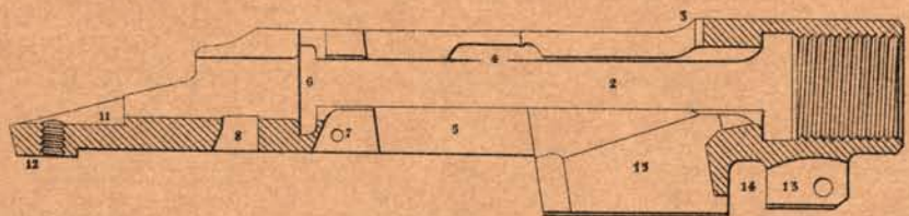
Fig.14. Coupe longitudinale.
