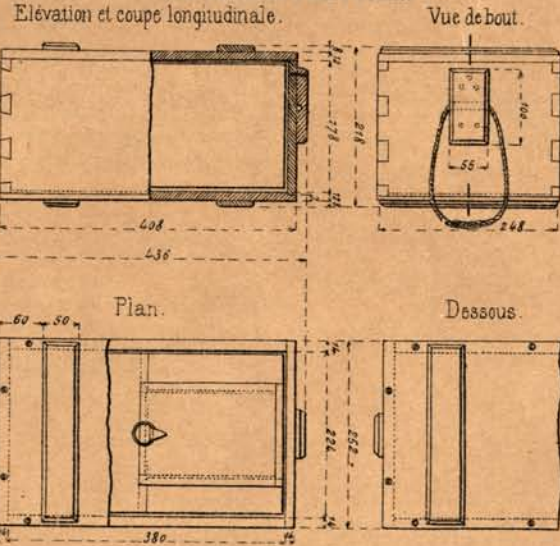
Fig. 7. Caisse C.1 bis avec caisse intérieure en zinc. Elevation et coupe longitudinale. Vue de bout.
