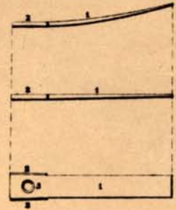
Fig 12 Ressort de hausse
