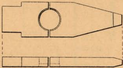
Fig. 4. Etampes pour resserrer la poignée. (1/2).
