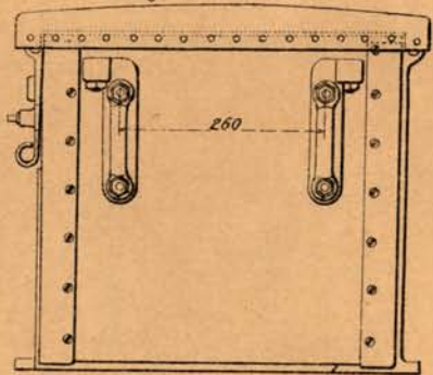
Fig. 2. Vue de bout.
