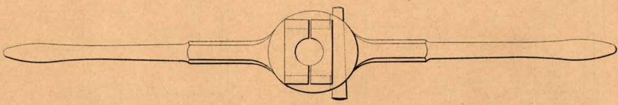
Fig. 2. Coussinets de tourne à gauche: pour canons de carabine et de mousqueton. ( \frac{1}{2} )
